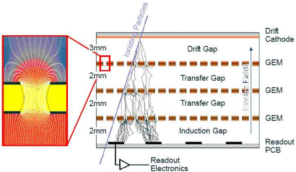
FIG. 2.5: Principe de fonctionnement d'un détecteur GEM.
