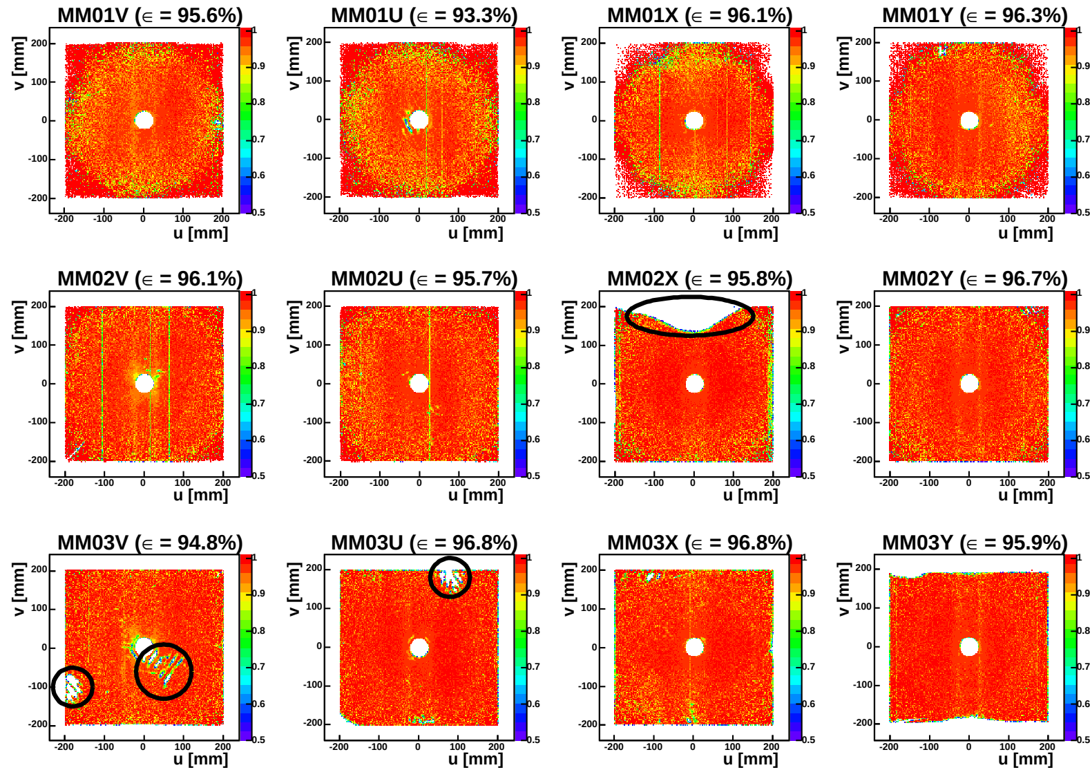
FIG. 4.4: Efficacités en deux dimensions pour les 12 plans de Micromegas en 2004. Les principaux défauts locaux ont été entourés. L'effet sur l'efficacité moyenne n'est pas significatif, sauf dans le cas de MM03V.
