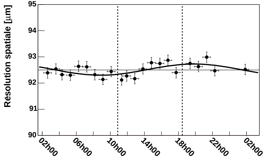
FIG. 4.8: Résolution spatiale moyenne des 12 plans de Micromegas au cours de la journée du 13 juillet 2004. Les lignes en pointillés indiquent les renversements de champ du solénoïde; la ligne horizontale correspond à la résolution moyenne. La fonction utilisée pour l'ajustement est de la forme de l'équation 4.1.
