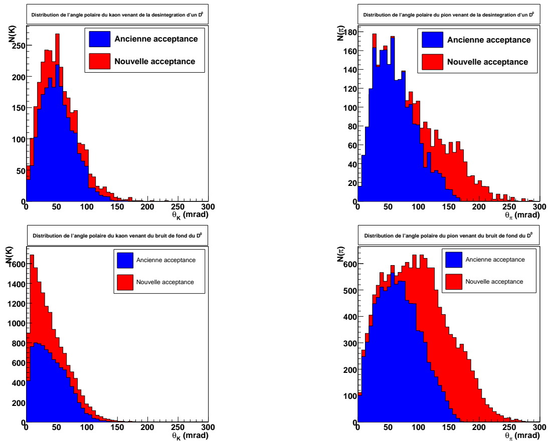
FIG. 3.15: Distribution angulaire des kaons (à gauche) et des pions (à droite) provenant d'un méson D^0 (en haut) ou du bruit de fond (en bas) associée à l'ancienne et à la nouvelle acceptation de l'aimant de la cible. Ces histogrammes sont obtenus à partir des données 2006 pour lesquelles l'ancienne acceptation a été artificiellement appliquée.
