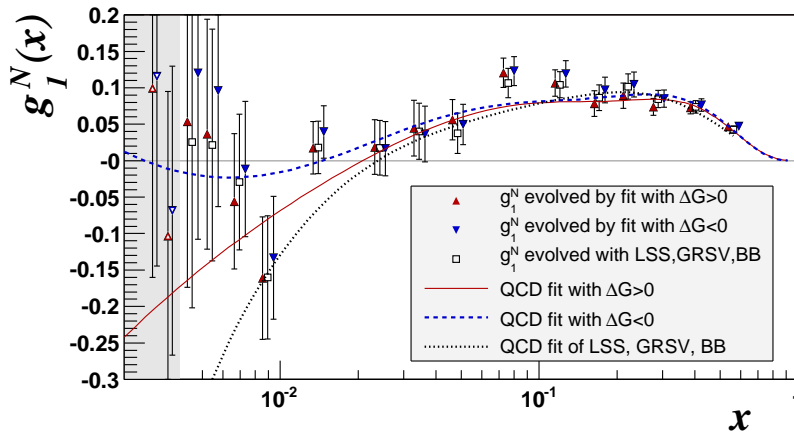
FIG. 1.5: Les données de g_1 mesurées par l'expérience COMPASS sont ajustées par une paramétrisation. Deux solutions correspondant à \Delta G > 0 et \Delta G < 0 sont équivalentes.
