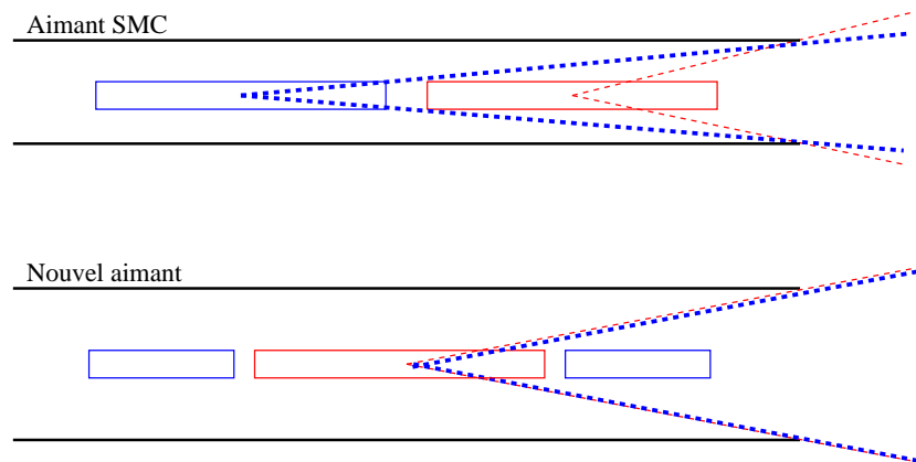
FIG. 3.16: Dispositifs de la cible avec l'aimant SMC (haut) pour les années 2002-2004 et avec le nouvel aimant (bas) pour les années suivantes. La configuration à trois cellules permet une acceptation équivalente pour les deux états de spin (bleu et rouge).
