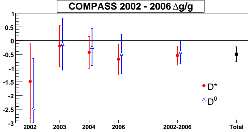
FIG. 6.1: \Delta g/g mesuré pour chaque année et pour les canaux D^0 et D^* . Ces résultats sont ensuite regroupés sur les quatre années 2002-2006 puis combinés pour les deux canaux.
