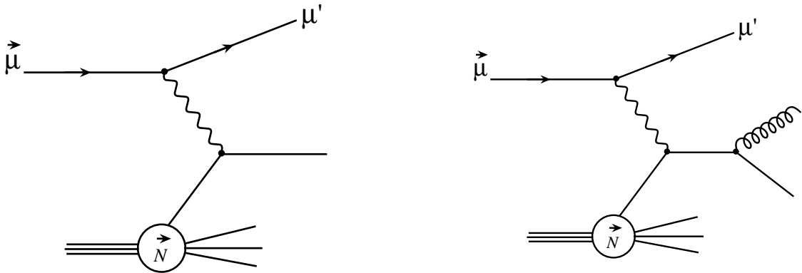
FIG. 2.2: Processus concurrents du PGF. A gauche : processus DIS à l'ordre 0 (LO). A droite : processus QCD Compton (QCDC).
